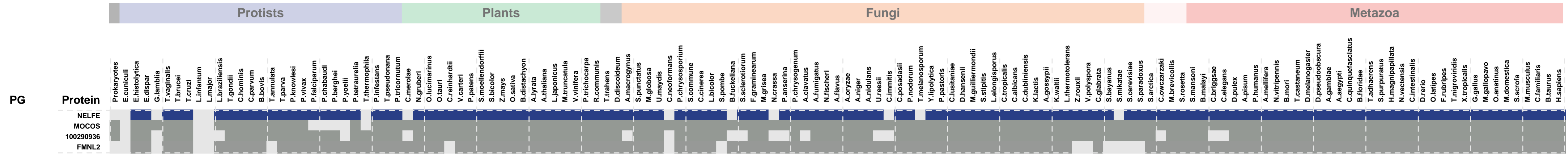
1: NELF complex
